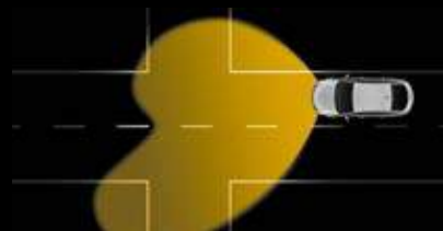
7. En ville. Faisceau de lumière plus large et abaissé. Sensible à la vitesse du véhicule et à l'éclairage urbain.
